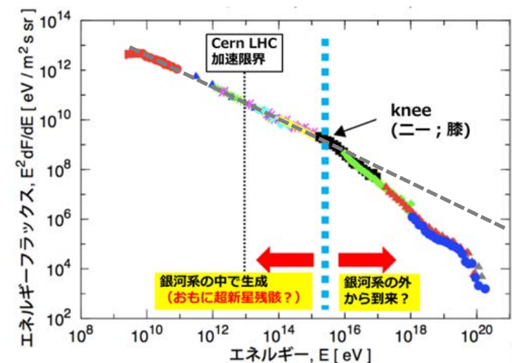
図 1：宇宙線スペクトルの概観と「knee」
