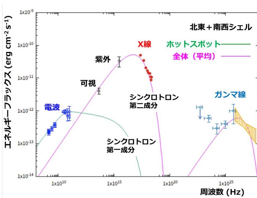
図 5 : SN1006 の電波からガンマ線にわたる多波長スペクトル。電波と X 線はシンクロトロン放射と考えられるが、別の成分で滑らかにつながらないことが分かる
